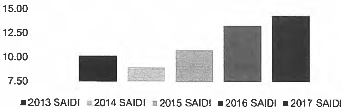
Gráfica 2: SAIDI - Puerto Rico (2013-2017)
